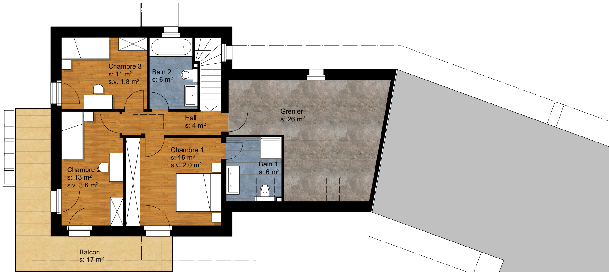
Villa 1 Étage
